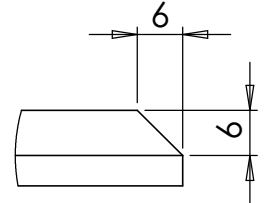
DÉTAIL A ECHELLE 1 : 1
